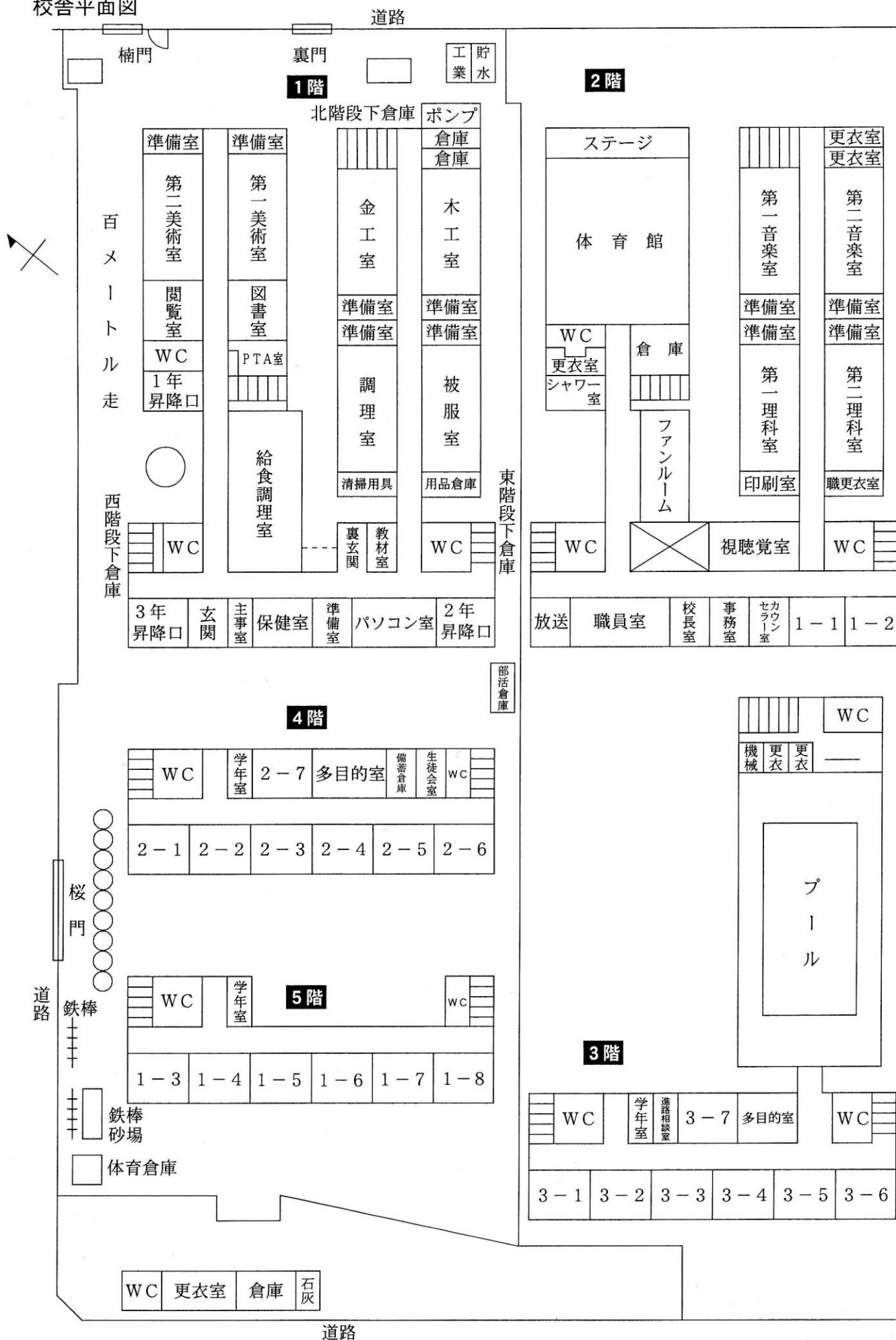
校舎平面図
